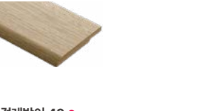
걸레받이 40 ● · 소재 MDF · 규격 40(W) × 2,400(H) × 9(T)
