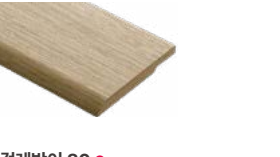
걸레받이 80 ● · 소재 MDF · 규격 80(W) × 2,400(H) × 9(T)
