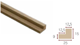
마이너스 몰딩 25 · 소재 MDF · 규격 25(W) × 2,400(H) × 15(T) · 가능 한샘 100, S200
