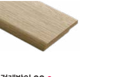
걸레받이 60 ● · 소재 MDF · 규격 60(W) × 2,400(H) × 9(T)
