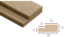
2계단 몰딩 · 소재 MDF · 규격 50(W) × 2,400(H) × 12(T)
